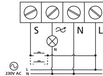
Kopplingschema
